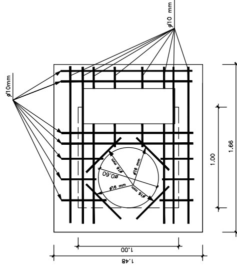
DISTRIBUCION DE LA ARMADURA DE LA LOSA
