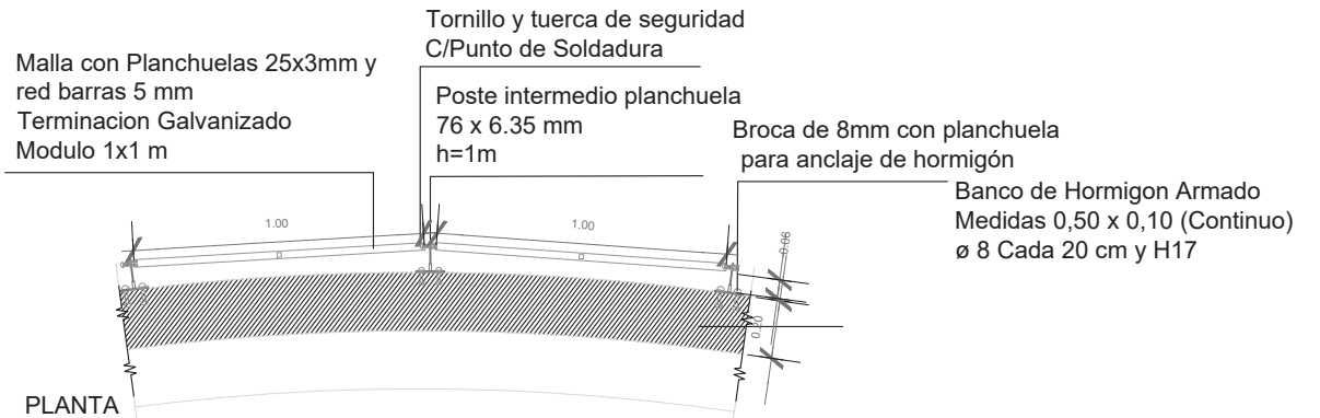
PLANTA
