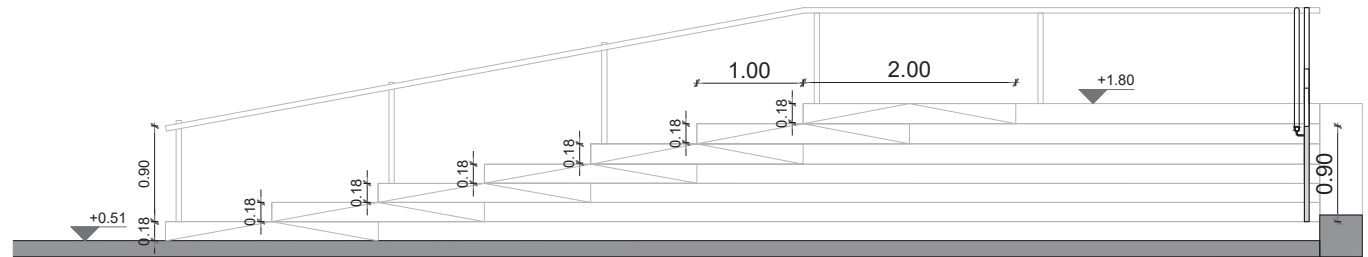
VISTA LATERAL Esc.: 1:50
