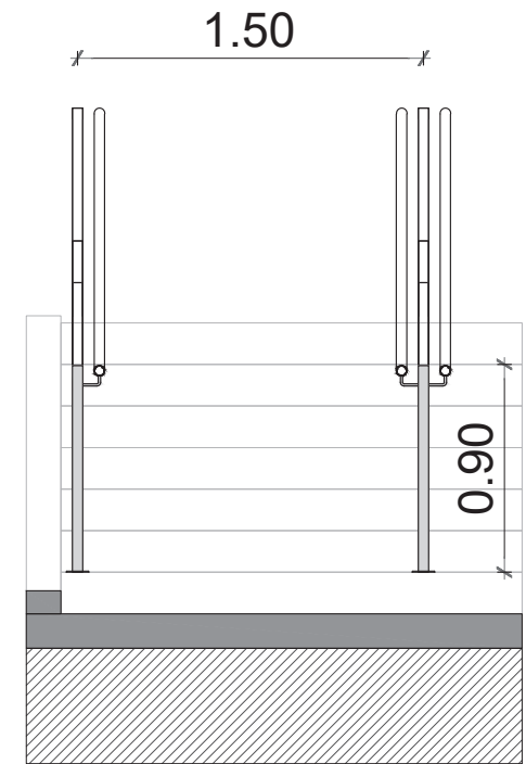
CORTE Esc.: 1:25
