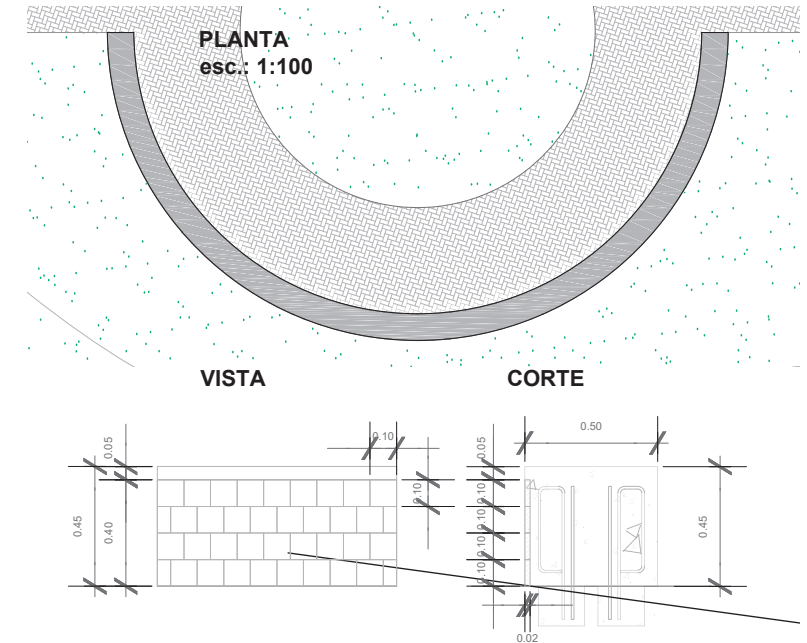
Banco circular de H°A° in situ esc.: 1:20
