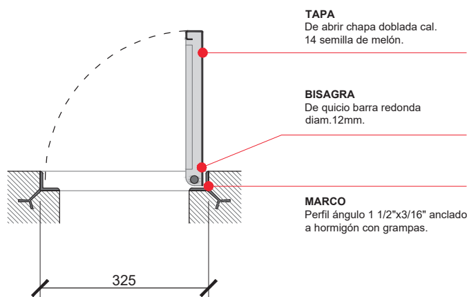
Corte transversal
