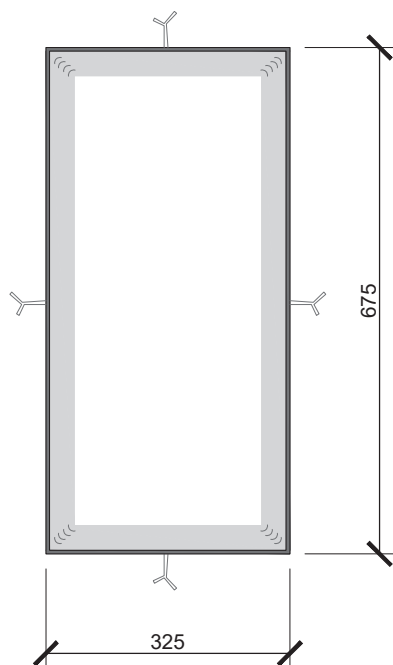
Planta Marco
