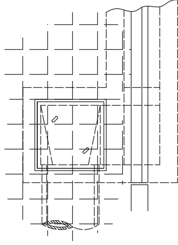
VARIANTE CON CAÑO DE SALIDA LATERAL
