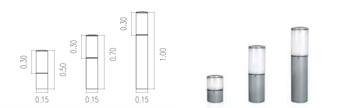
LUMINARIA ORNAMENTAL - TIPO LUCCIOLA BOLLARD LED
